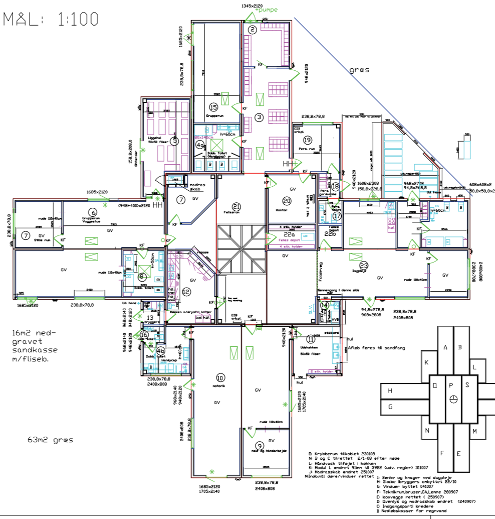
Grundrissplan eines Gebäudes mit grosse Flexibilität
